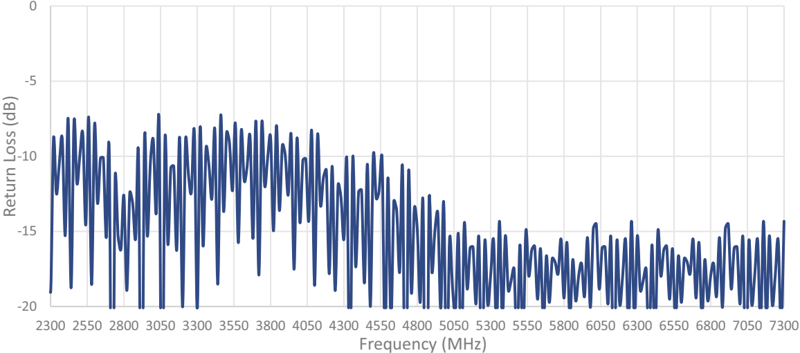
Cable 3: WIFI-6-6E
