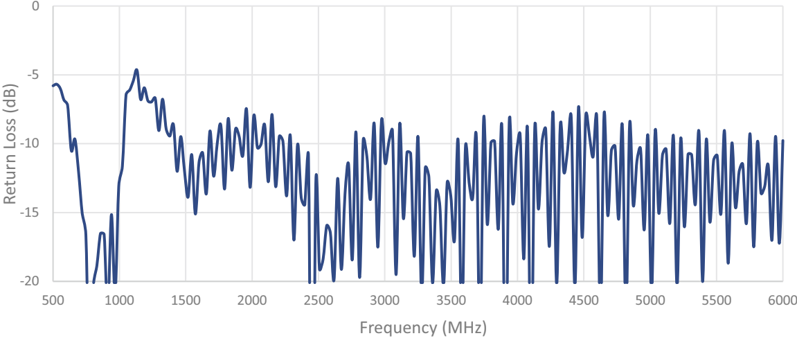
Cable 2: 5GNR
