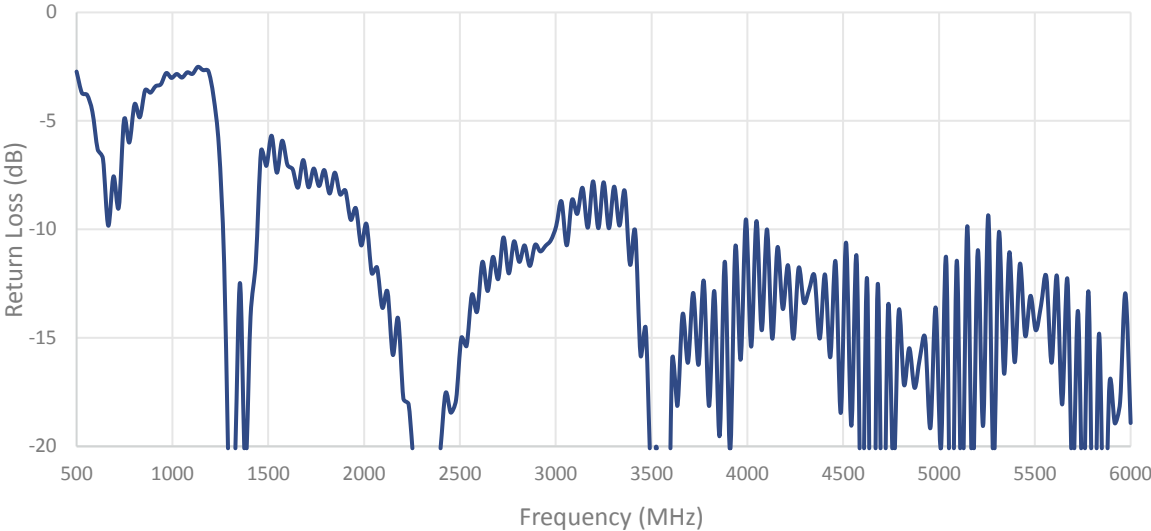
Cable 2: 5GNR
