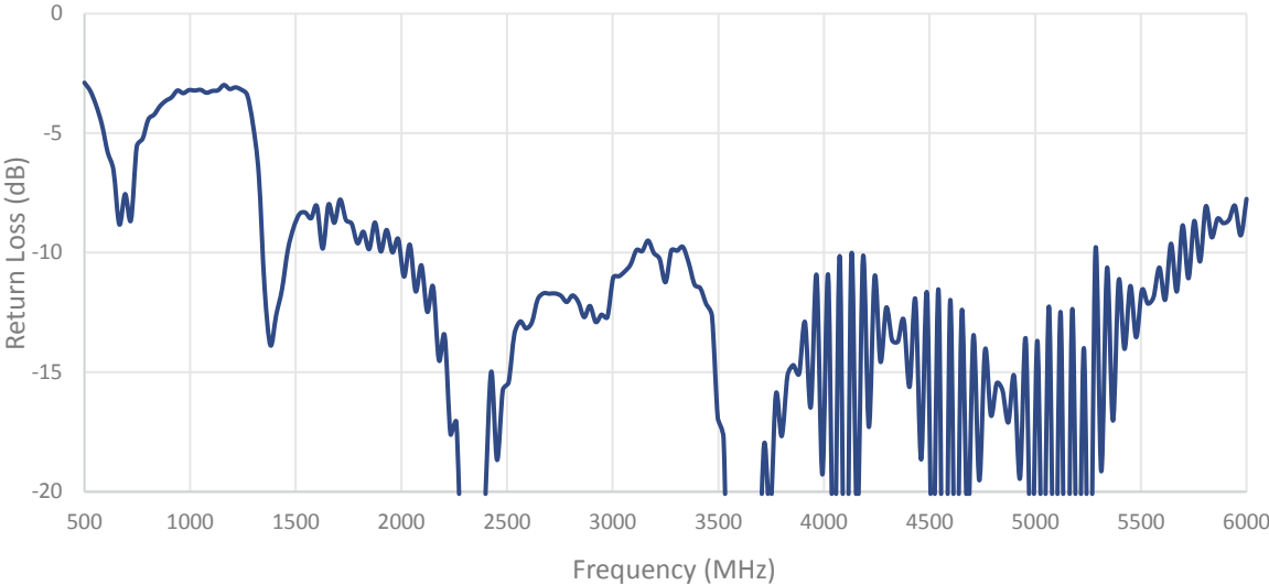
Cable 3: 5GNR
