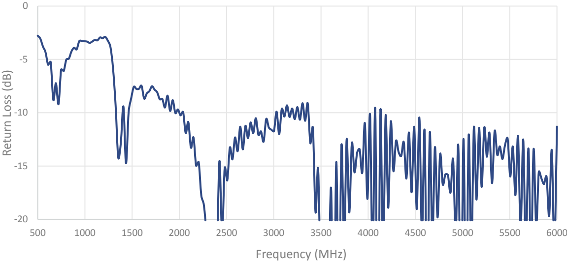
Cable 4: 5GNR
