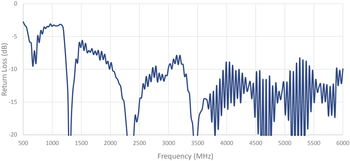
Cable 1: 5GNR
